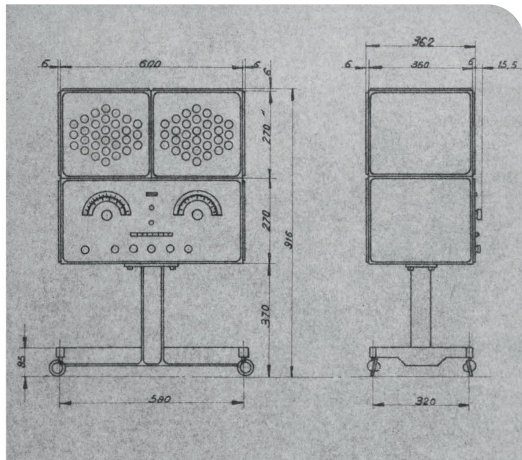
Disegni tecnici BRIONVEGA (1967)
